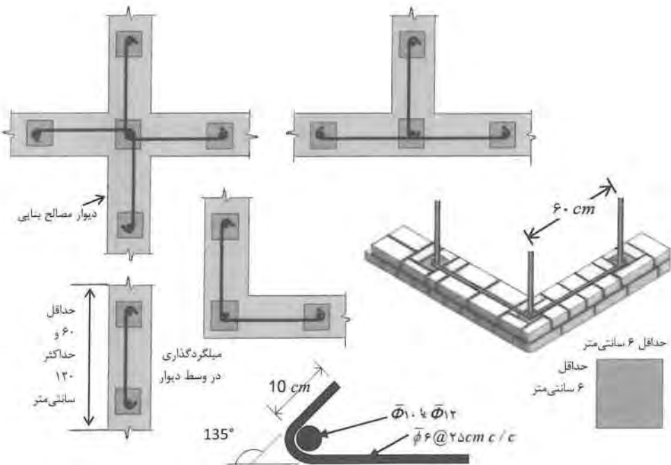
شکل ۷-۲ جزئیات میلگردهای قائم و افقی در سامانه میلگردگذاری معادل
