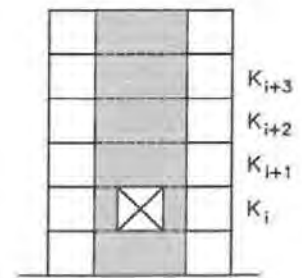
K_i < 0.6 K_{i+1} یا K_i < 0.7/3(K_{i+1} + K_{i+2} + K_{i+3})
