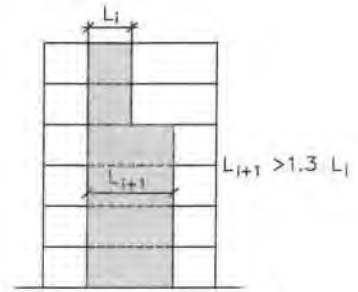
الف - نامنظمی هندسی
