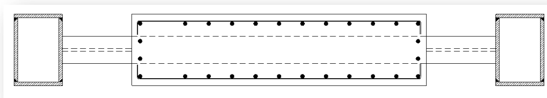
شکل (۳) ستون فولادی منفصل از دیوار
