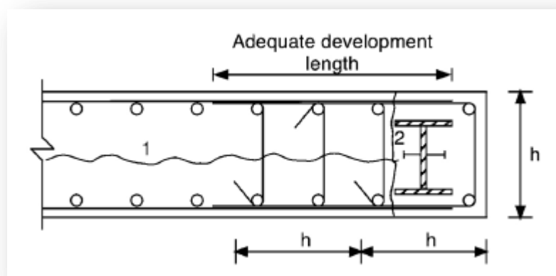
شکل (۷) مودهای شکافت محتمل بتن در اطراف ستون مدفون در دیوار برشی و میلگردهای مورد نیاز برای جلوگیری از آنها
