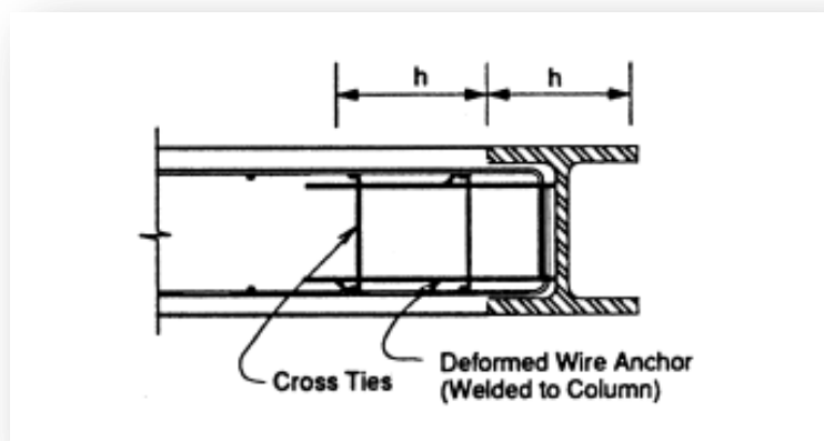
شکل (۲) ستون فولادی نیمه مدفون (و حداقل طول المان مرزی آن)
