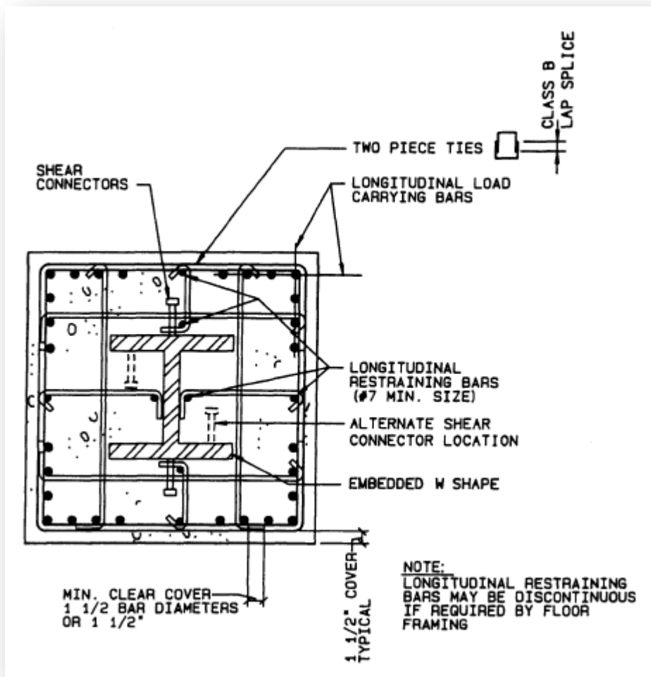
شکل (۴) مثالی از دیتایل‌های مناسب برای خاموت‌های اطراف ستون فولادی مدفون
