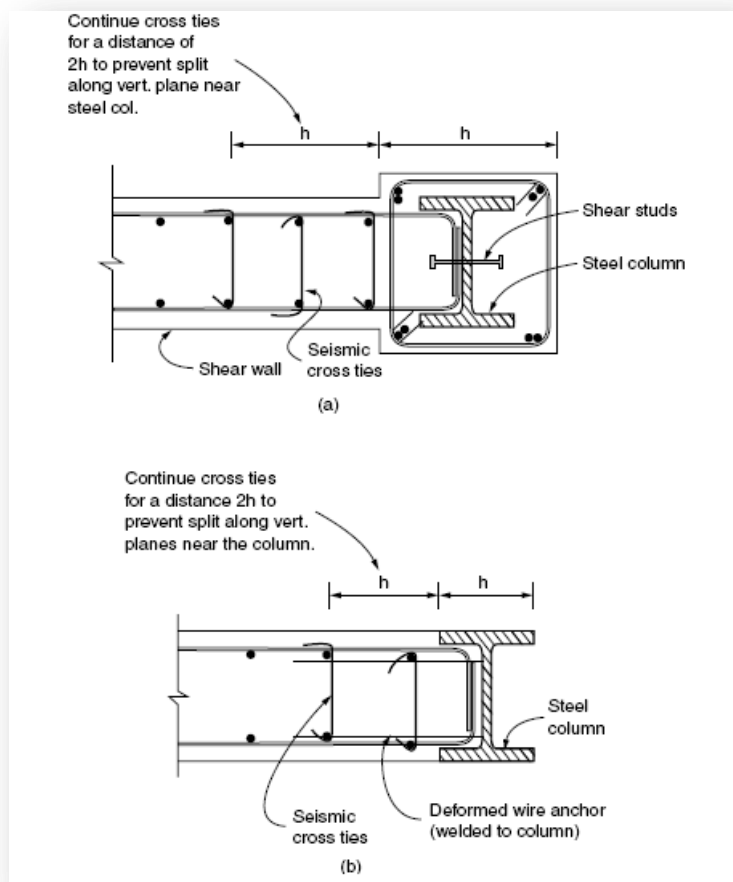
شکل (۸) المان مرزی دیوار برشی مرکب با ستون فولادی
