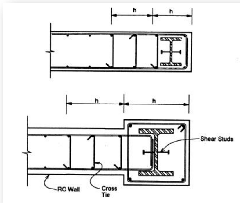
شکل (۱) ستون فولادی مدفون در دیوار برشی
