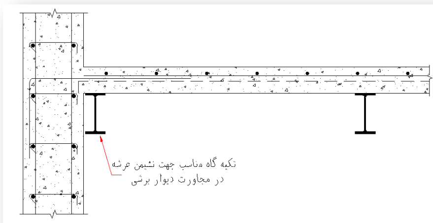
شکل (۱۳) تیرچه انتهایی نشیمن ورق های دوزنقه ای در سقف عرشه فولادی
